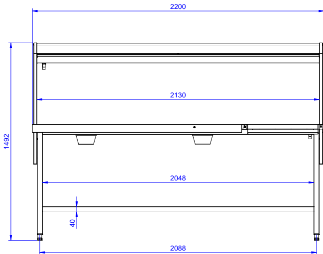
Front aanzicht
